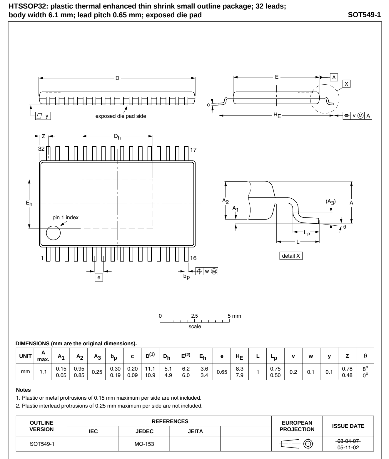
Fig 18. Package outline SOT549-1 (HTSSOP32)
